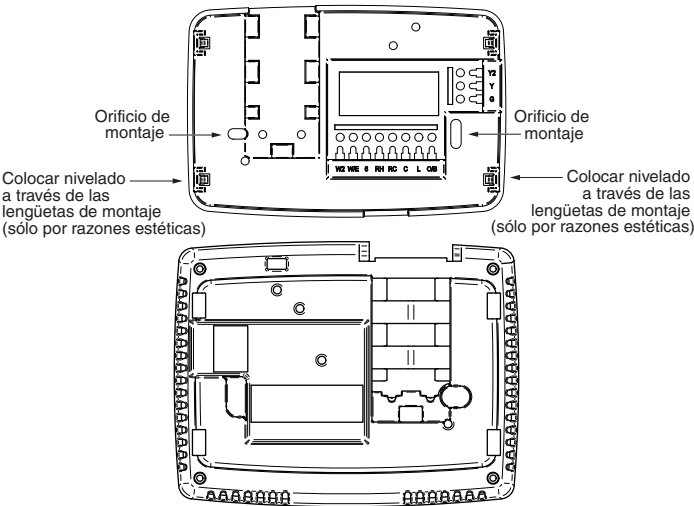
Figura 2 – Base del termostato y vista trasera del termostato
